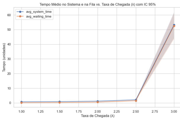
Figura 4: Tempo médio de espera ( W_q ) em função da taxa de chegada \lambda .
